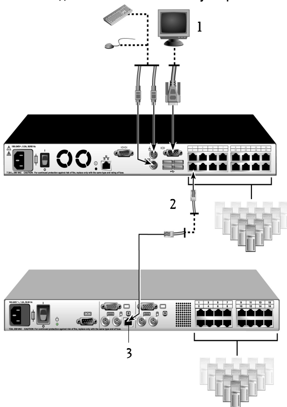
Рис. 2-12. Удаленный консольный коммутатор с аналоговым коммутатором CAT 5
